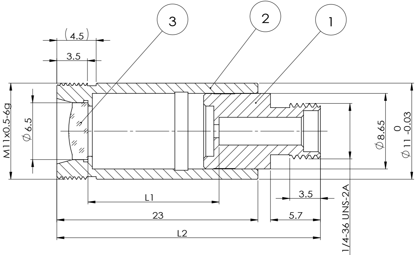
SECTION A-A
